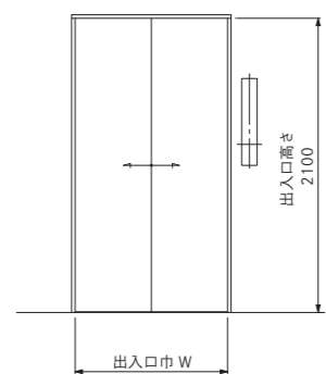
出入口正面図
